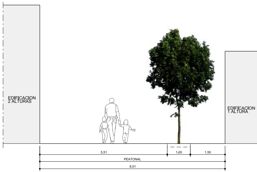
SECCIÓN I-I'
