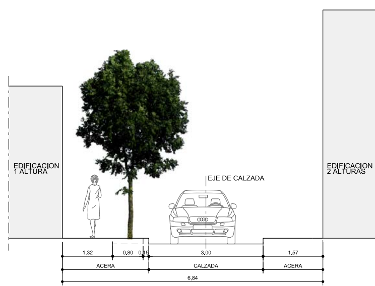
SECCIÓN J-J'
