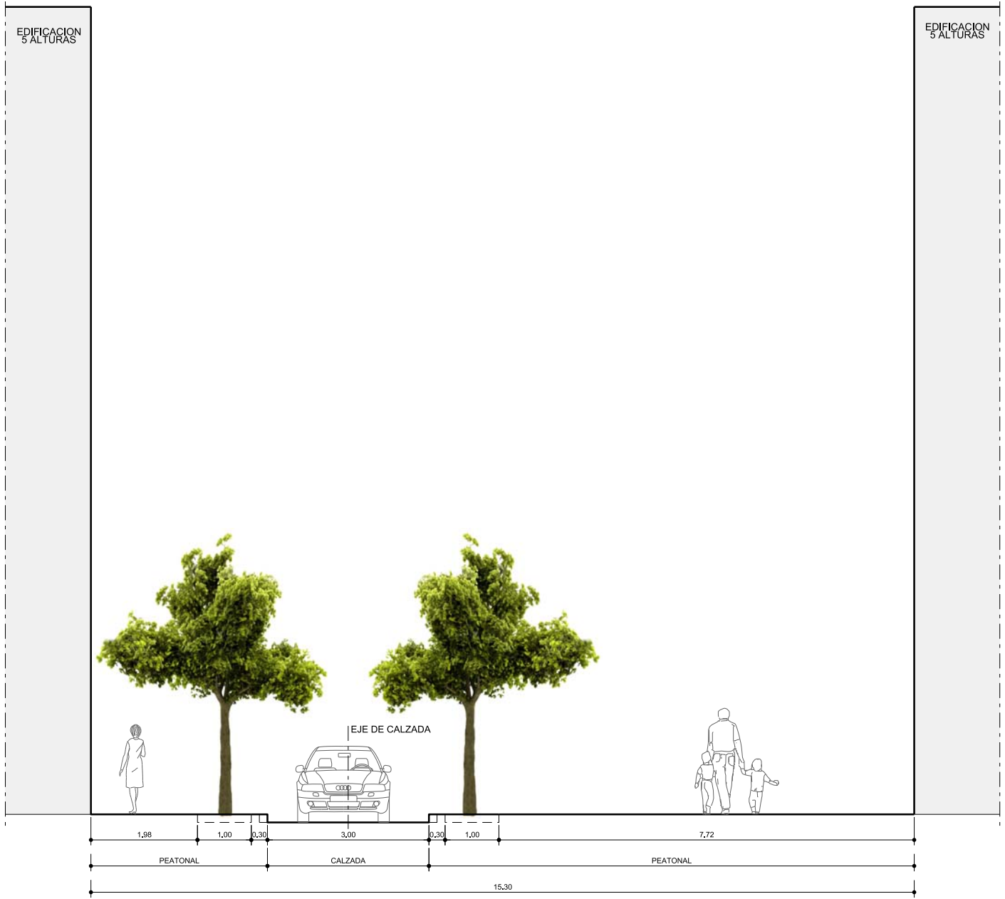
SECCIÓN C-C' (Calle La Rosa)
