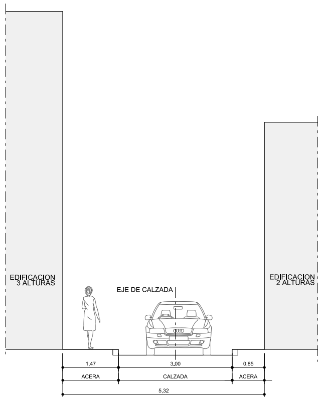
SECCIÓN K-K'
