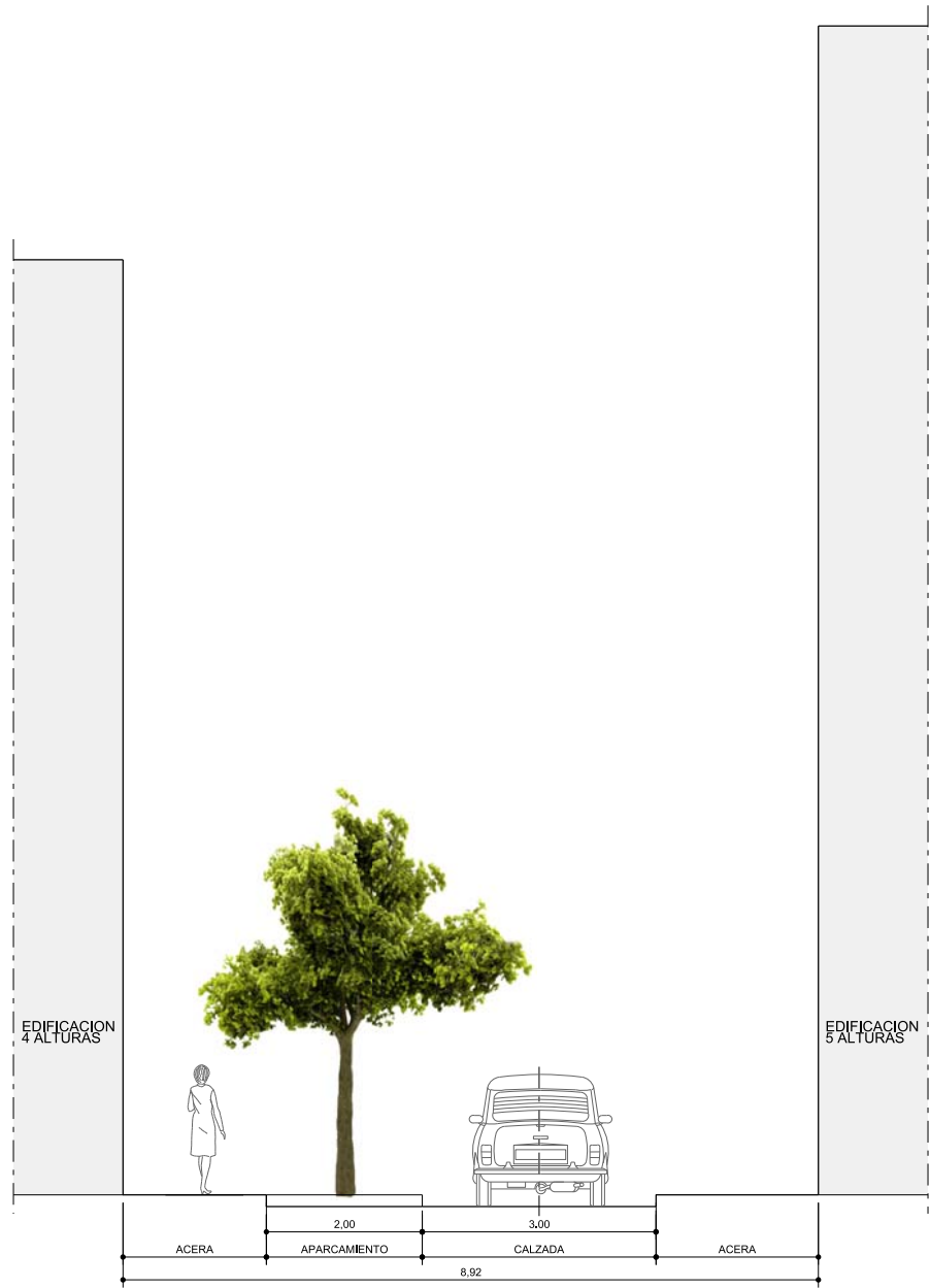
SECCIÓN H-H'
