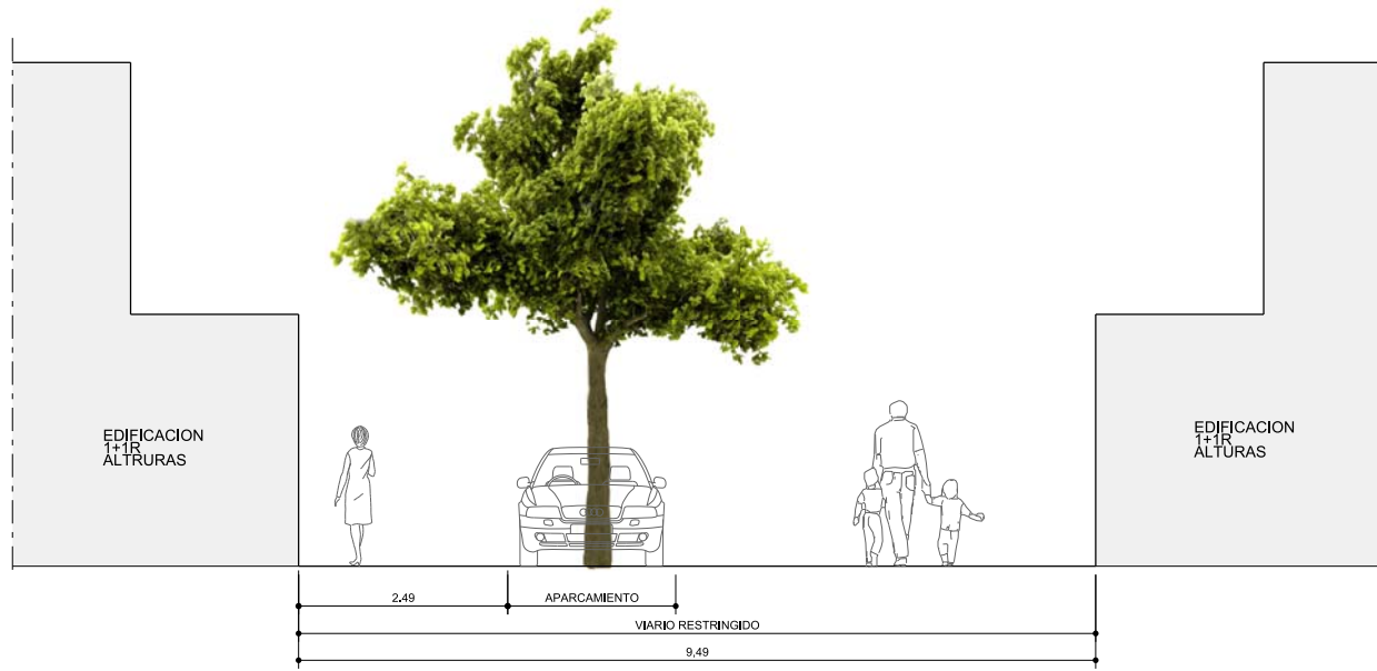
SECCIÓN M-M'
