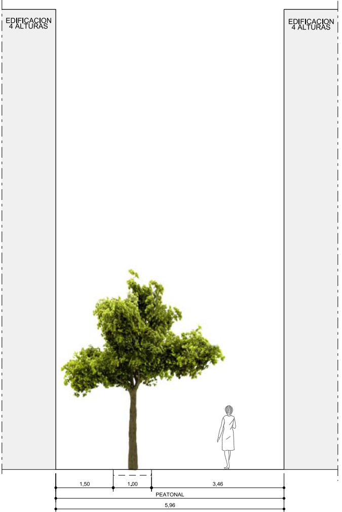
SECCIÓN G-G' (Calle San Miguel)
