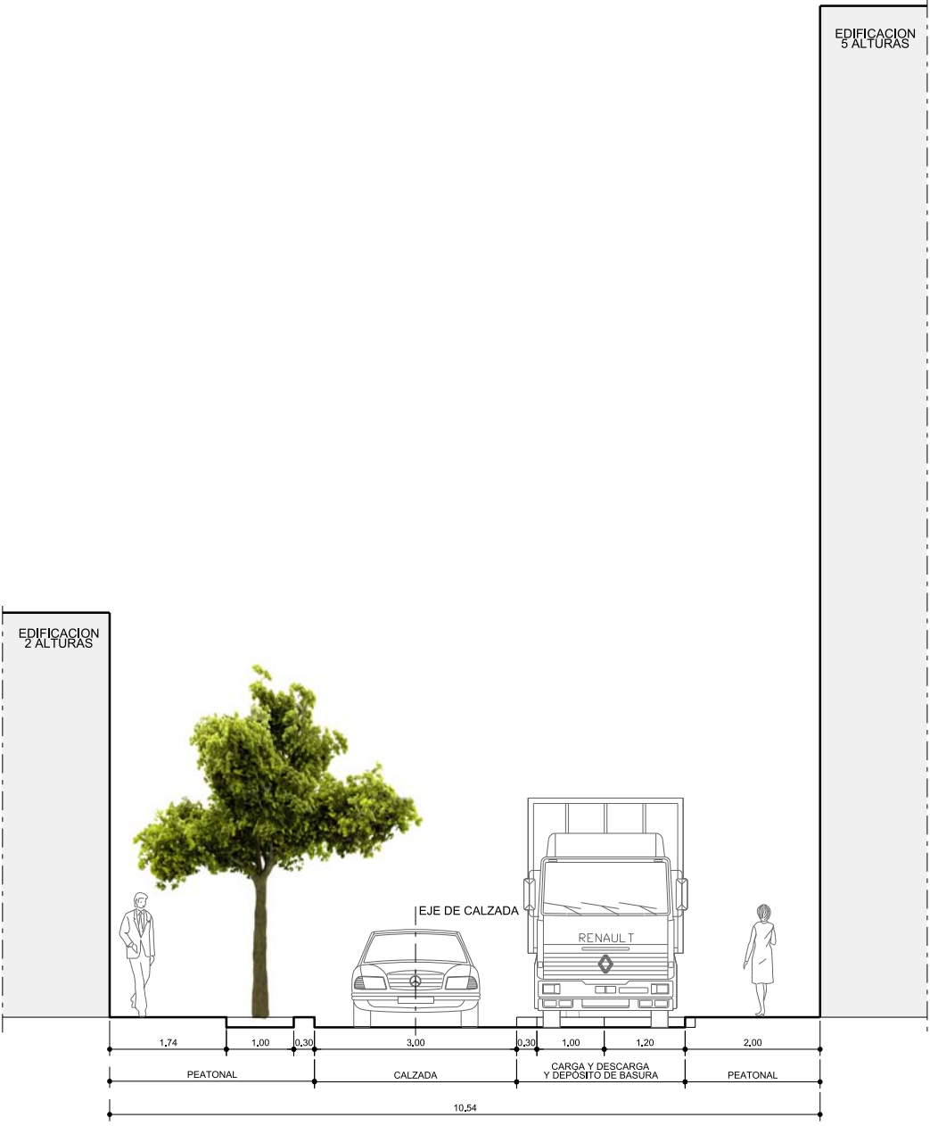
SECCIÓN B-B' (Calle La Rosa)
