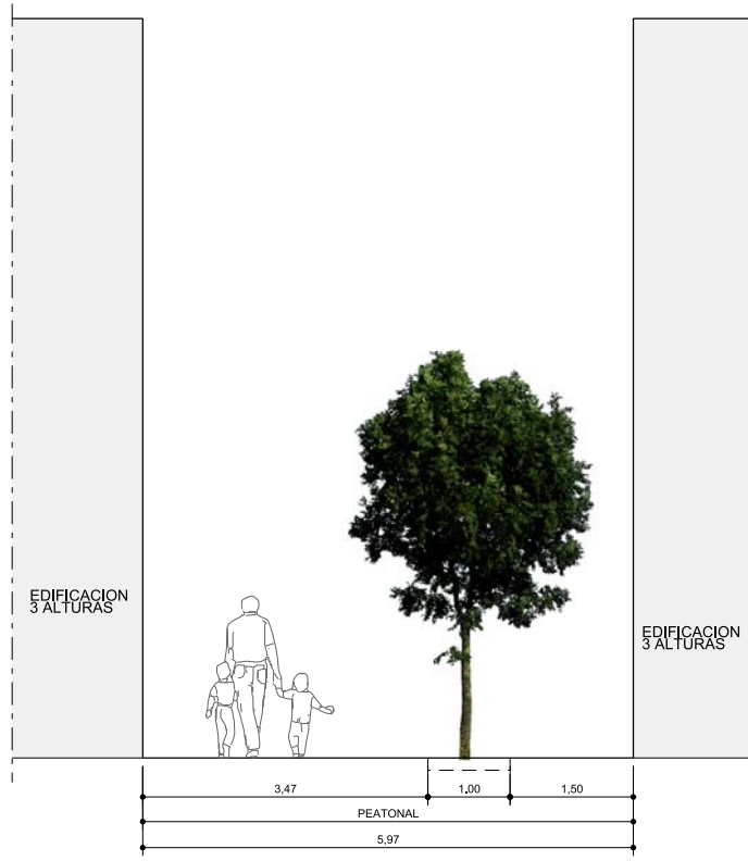
SECCIÓN L-L'
